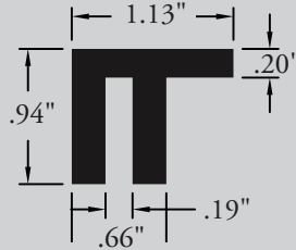
PS-567 1\" BAR-CLIP
