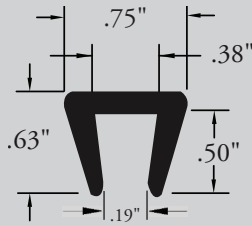
PS-567 1\" BAR-CLIP
